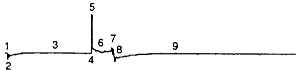
動力行程點火波形
