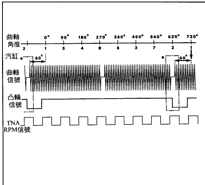
◎119(八缸)引擎波形：
