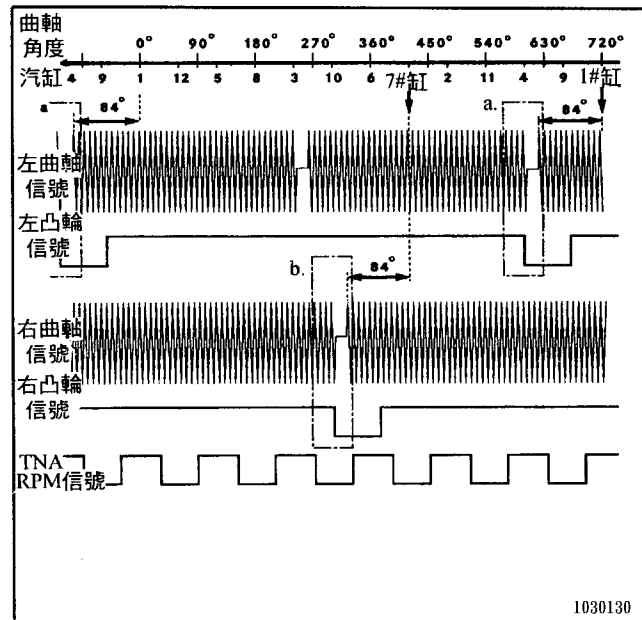
◎120(十二缸)引擎波形
