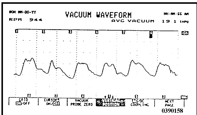
◎六缸引擎標準真空波形
