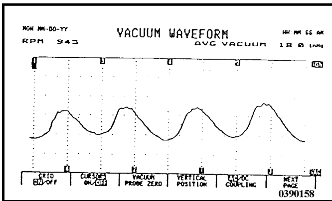
◎四缸引擎標準真空波形
