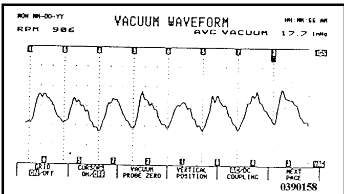
◎八缸引擎標準真空波形
