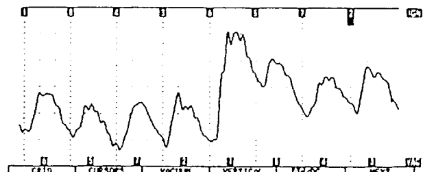
◎第一缸排氣門凸輪磨損
