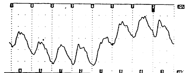
◎第一缸排氣門彈簧彈力太弱
