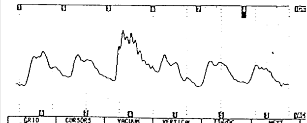
◎第四缸排氣門間歇調整太大
