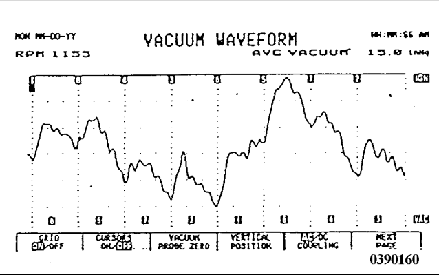
◎第五缸進氣門嚴重漏氣
