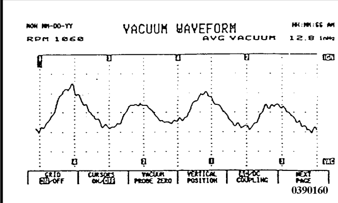
◎第四缸進氣門輕微漏氣
