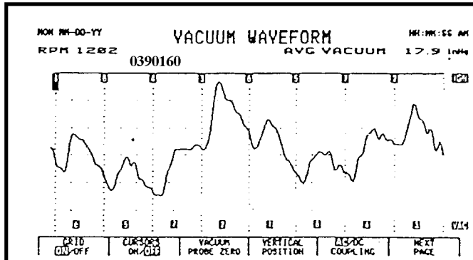
◎第三缸進氣門輕微漏氣
