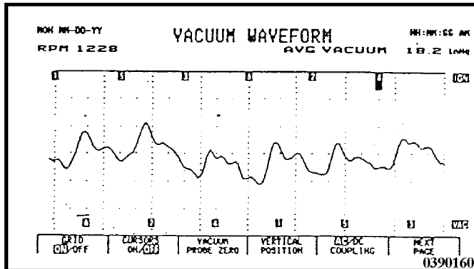
◎第二缸進氣門輕微漏氣
