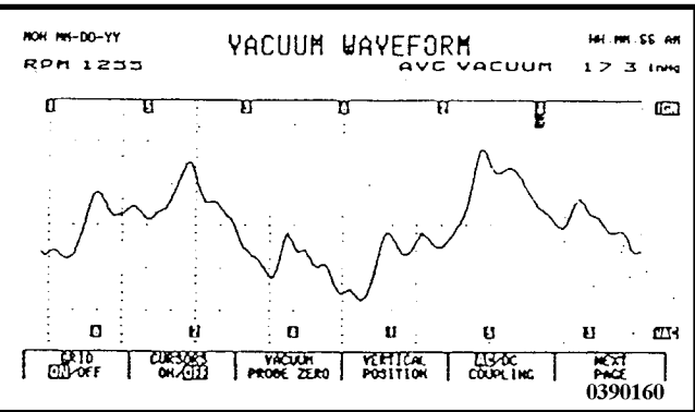
◎第二缸進氣門嚴重漏氣
