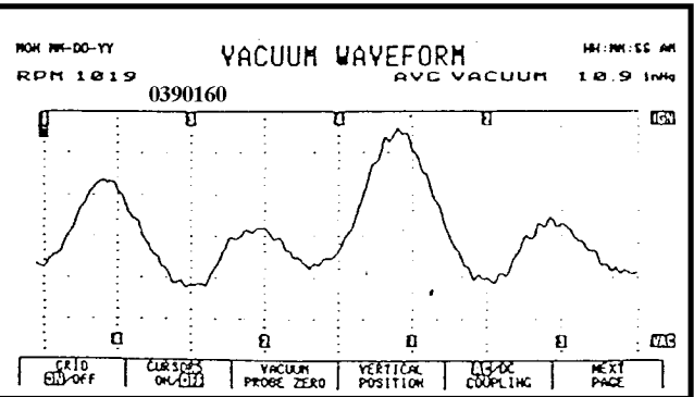
◎第四缸進氣門嚴重漏氣
