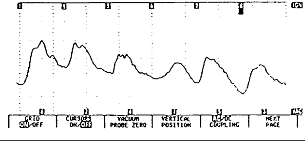
◎第一缸汽門推桿彎曲
