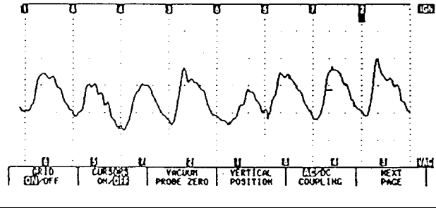
◎第一缸進氣門凸輪磨損
