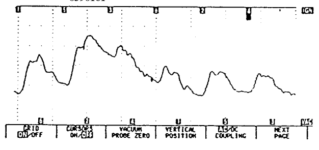
◎第二缸活塞環端間隙沒有錯開
