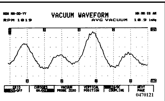
第四缸主進氣門漏氣
