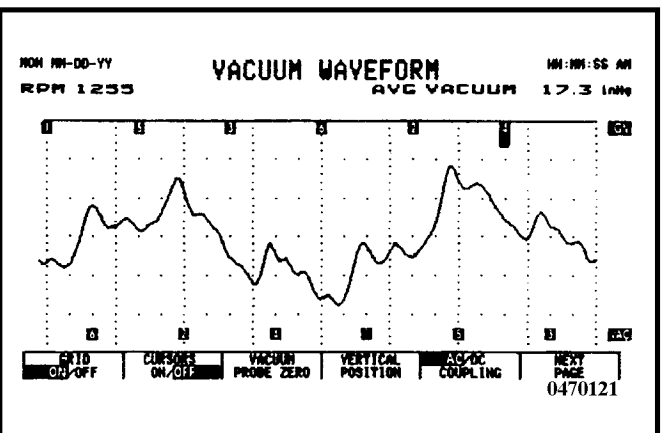
第二缸主進氣門漏氣
