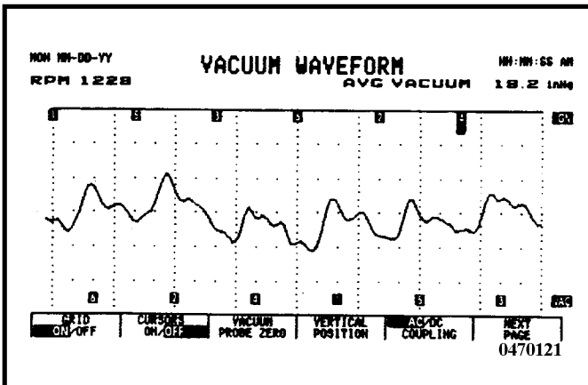
第二缸副進氣門漏氣
