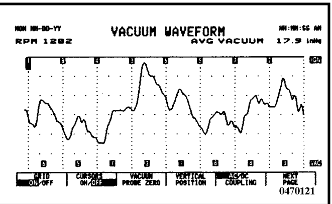
第三缸主進氣門漏氣
