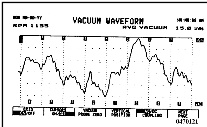
第五缸主進氣門漏氣
